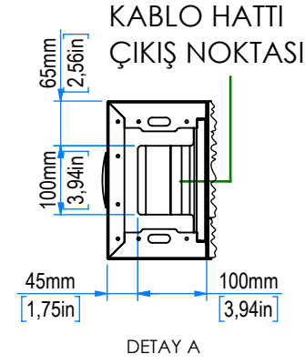
DETAY A
